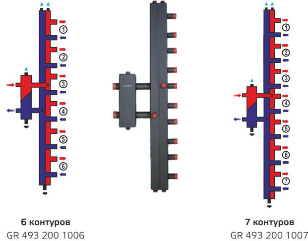
Гидравлический коллектор универсальный вертикальный, до 70 кВт
