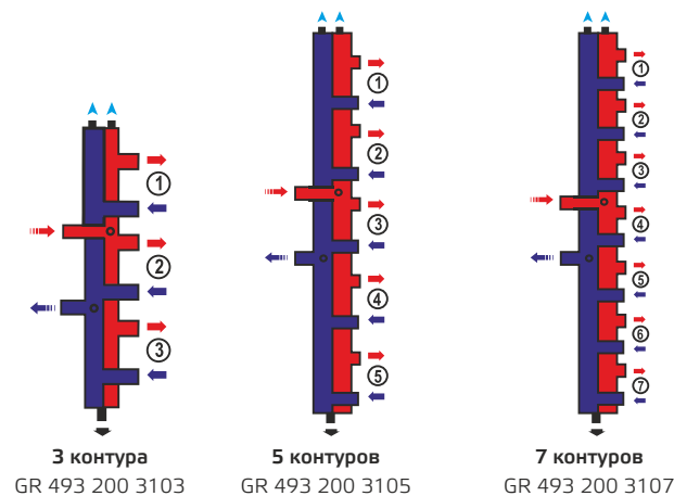
Гидравлический коллектор универсальный вертикальный, до 70 кВт
