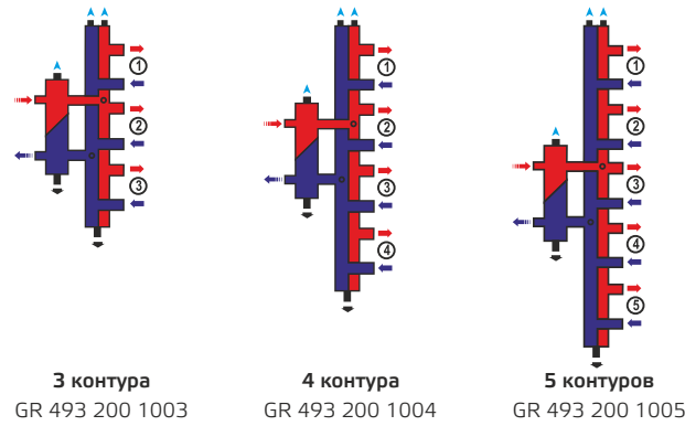
Гидроразделитель с коллектором вертикальный, до 70 кВт
