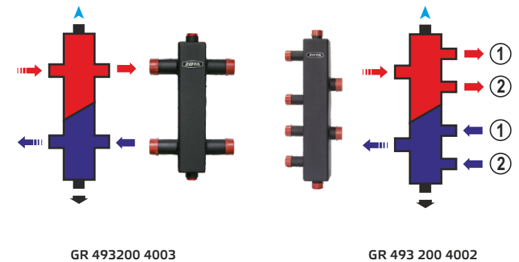
Гидроразделитель универсальный, до 50 кВт Гидроразделитель универсальный вертикальный 2 контура, до 50 кВт
