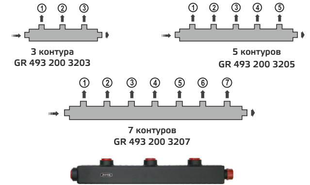
Гидравлический коллектор универсальный горизонтальный, до 70 кВт
