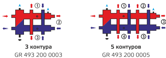
Гидроразделитель с коллектором горизонтальный, до 70 кВт
